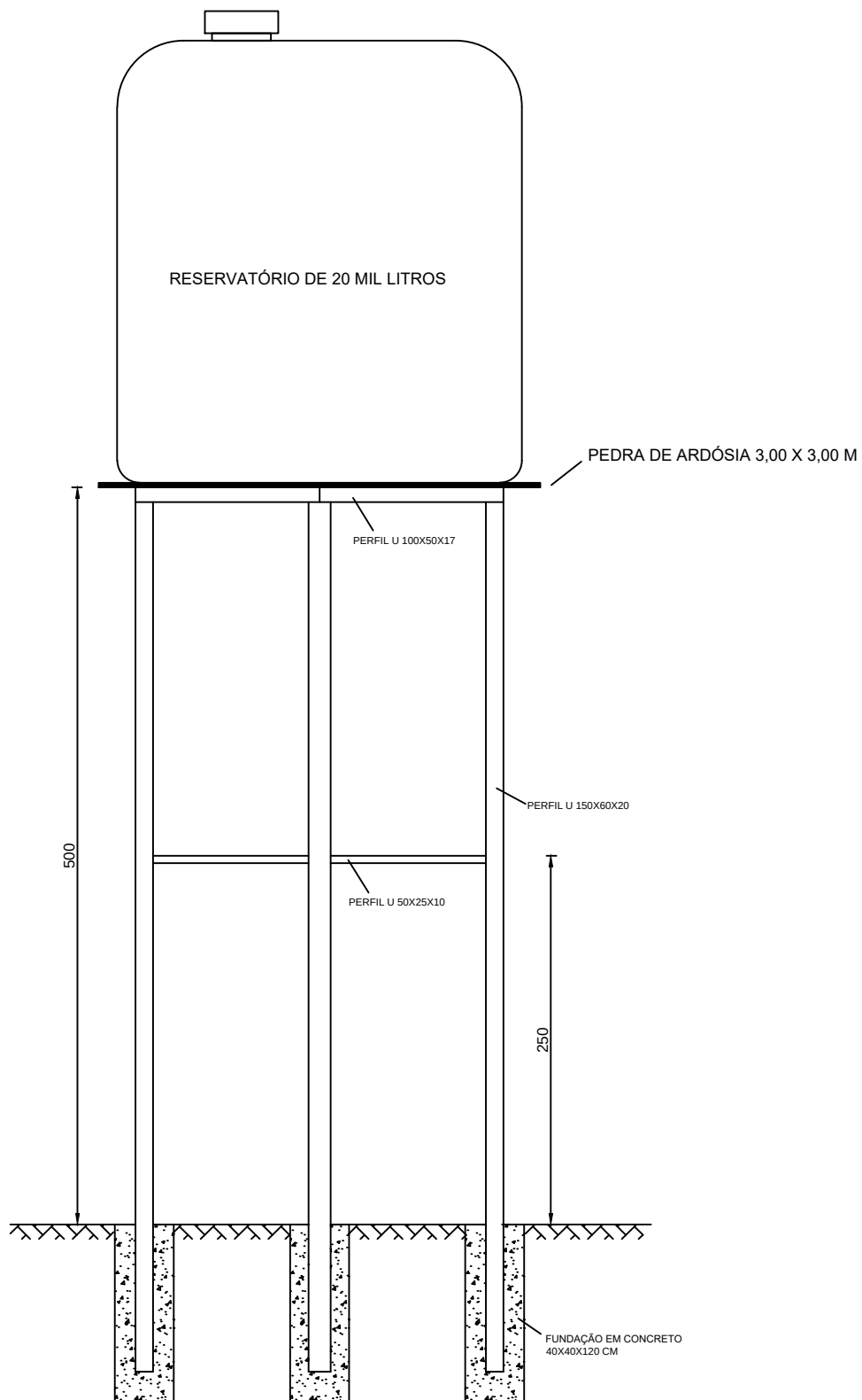
CORTE A-A
